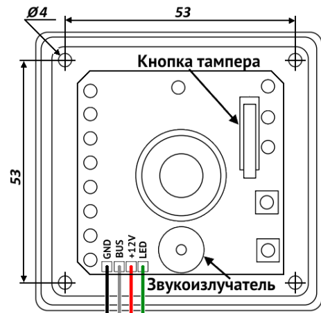
Рисунок 11. УИУ «Линд-11ТМ» без крышки
