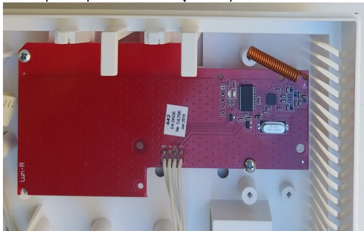
Рисунок 20. Радиоприемник "Lun-R" в корпусе прибора
