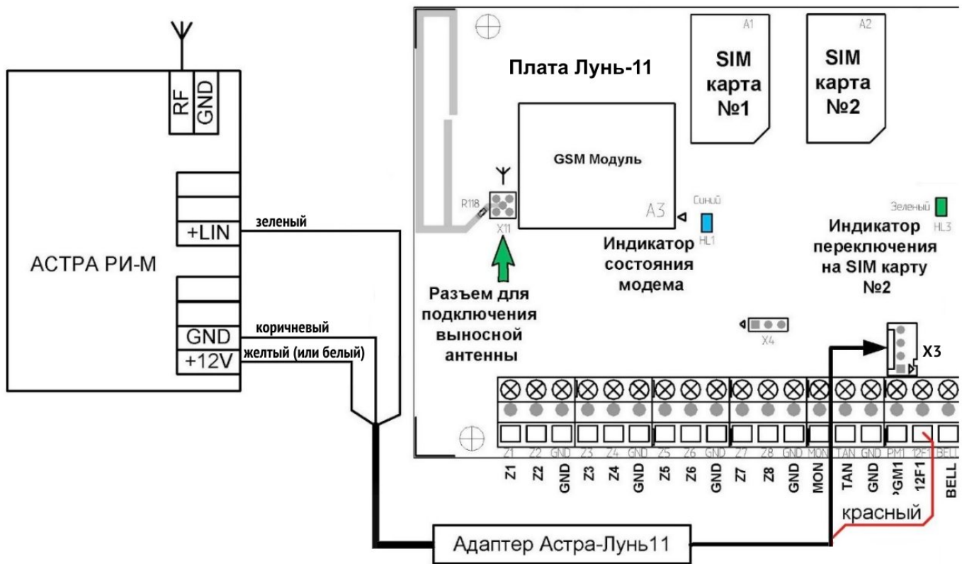
Рисунок 46. Схема подключения РПУ «Астра РИ-М»
