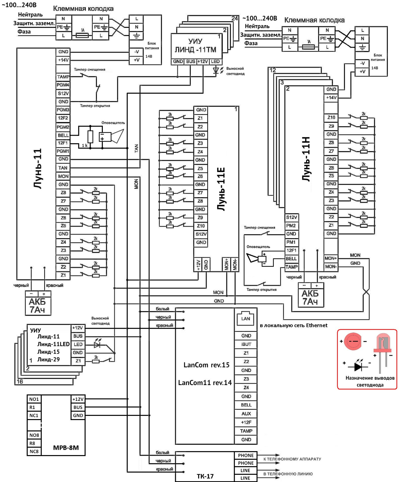
Рисунок 44. Схема подключения сетевых устройств
