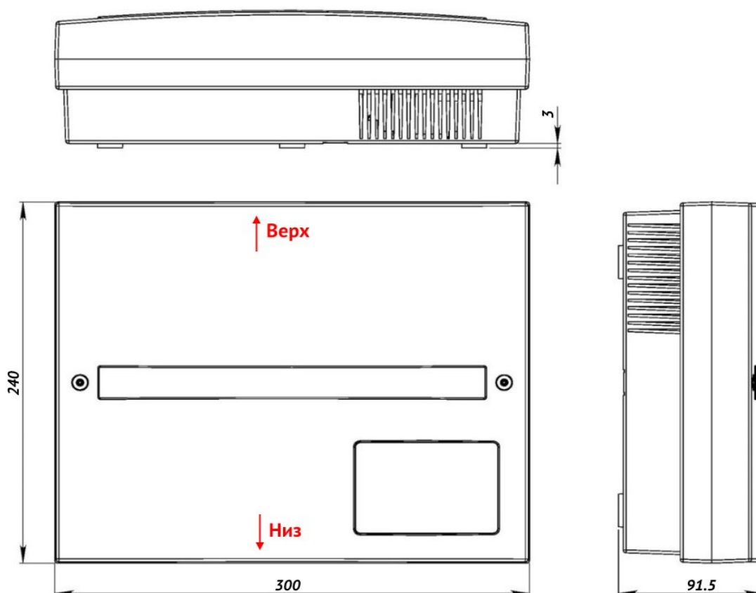
Рисунок 2. Габаритные размеры корпуса ППКОП
