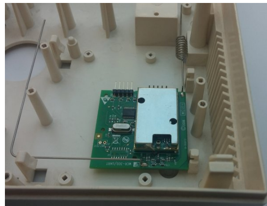
Рисунок 24. Радиоприемник «MCR-300» Visonic в корпусе прибора
