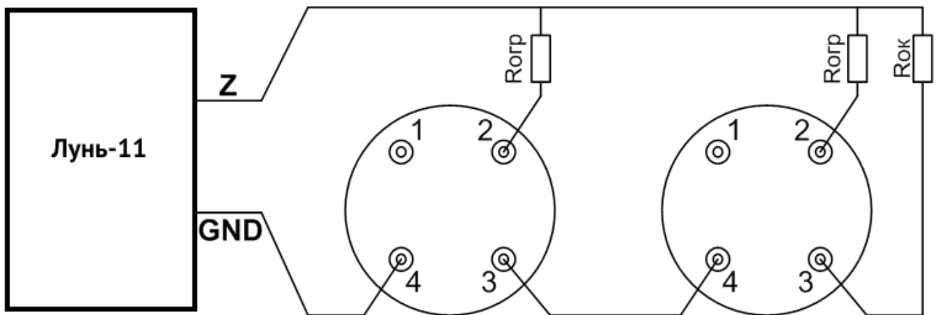
Рисунок 41. Схема подключения извещателей в пожарный шлейф по двухпроводной схеме
