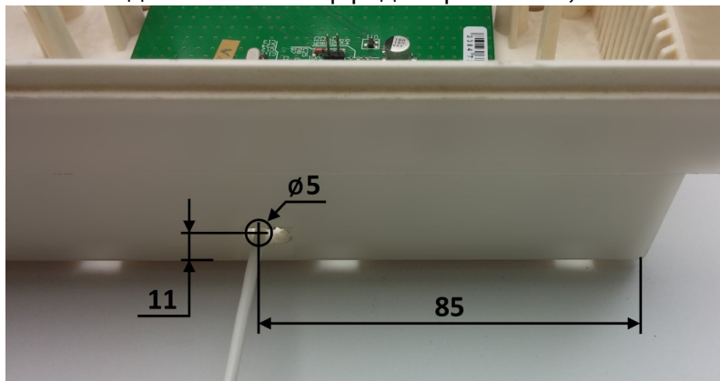
Рисунок 23. Отверстие в корпусе для антенны радиоприемника «P433» rev.4
