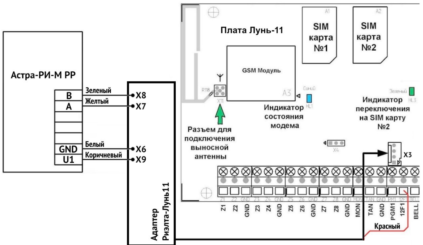
Рисунок 47. Схема подключения РПУ «Астра РИ-М РР»
