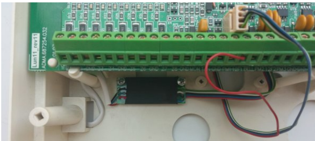
Рисунок 26. Установка и подключение адаптера «Астра-Лунь11»
