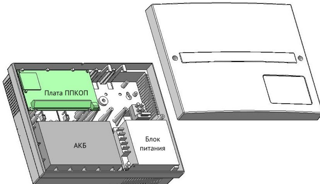
Рисунок 1. Размещение компонентов ППКОП в корпусе
