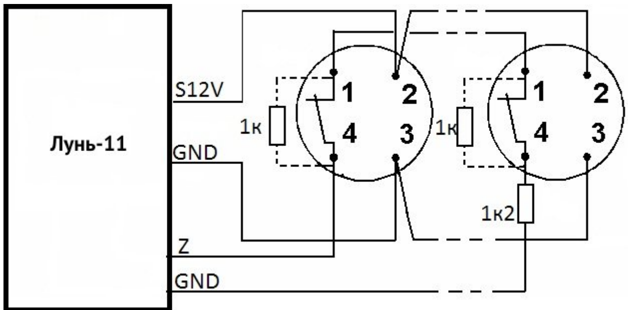
Рисунок 40. Схема подключения пожарных извещателей по четырехпроводной схеме
