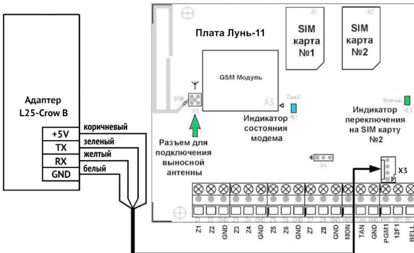
Рисунок 48. Схема подключения адаптера «L25-Crow B»
