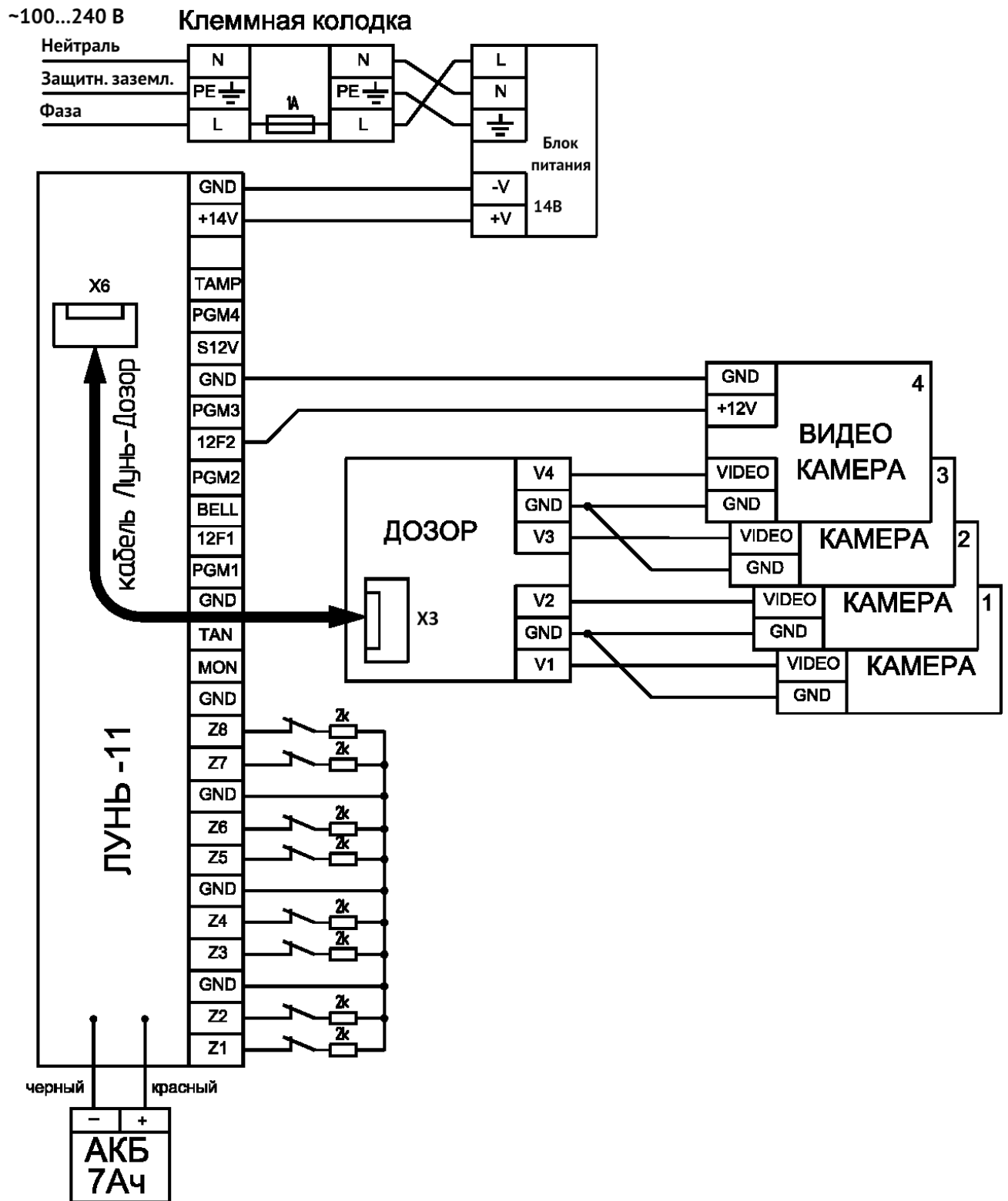
Рисунок 45. Схема подключения модуля фотоподтверждения тревог «Дозор»
