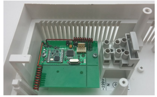
Рисунок 32. Радиоприемник Ajax «uartBridge» в корпусе прибора
