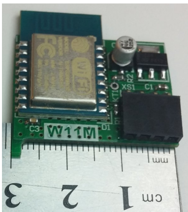
Рисунок 37. Общий вид модуля «W11M»
