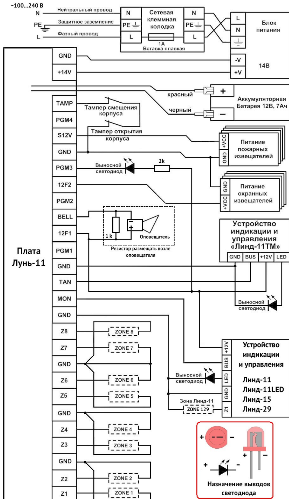
Рисунок 42. Схема подключения ППКОП
