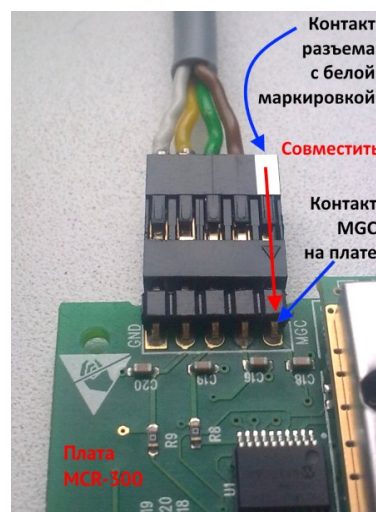
Рисунок 25. Подключение радиоприемника Visonic
