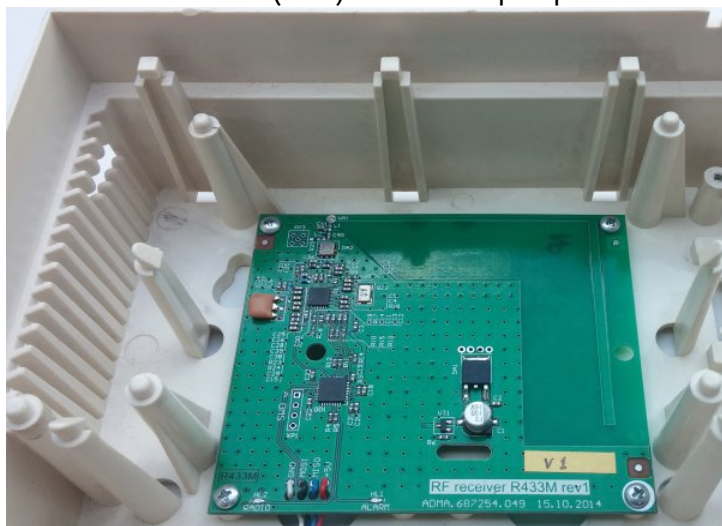
Рисунок 21. Радиоприемники серии «P433» в корпусе прибора
