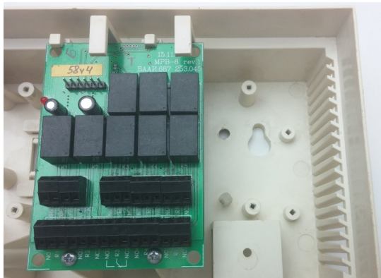
Рисунок 19. Модуль «MPB-8M» в корпусе прибора
