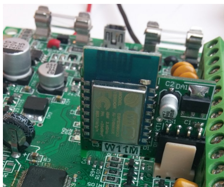
Рисунок 38. Установка модуля «W11M» в X3
